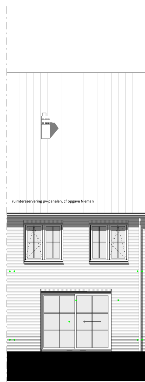
ACHTERGEVEL 1 : 100
