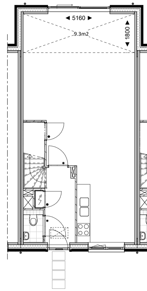
PLATTEGROND 1 : 100
