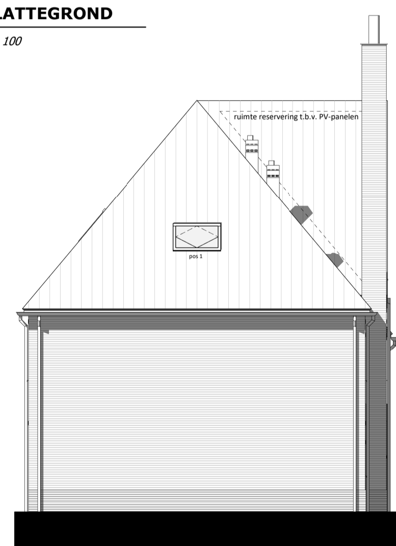
KOP GEVEL 1 : 100
