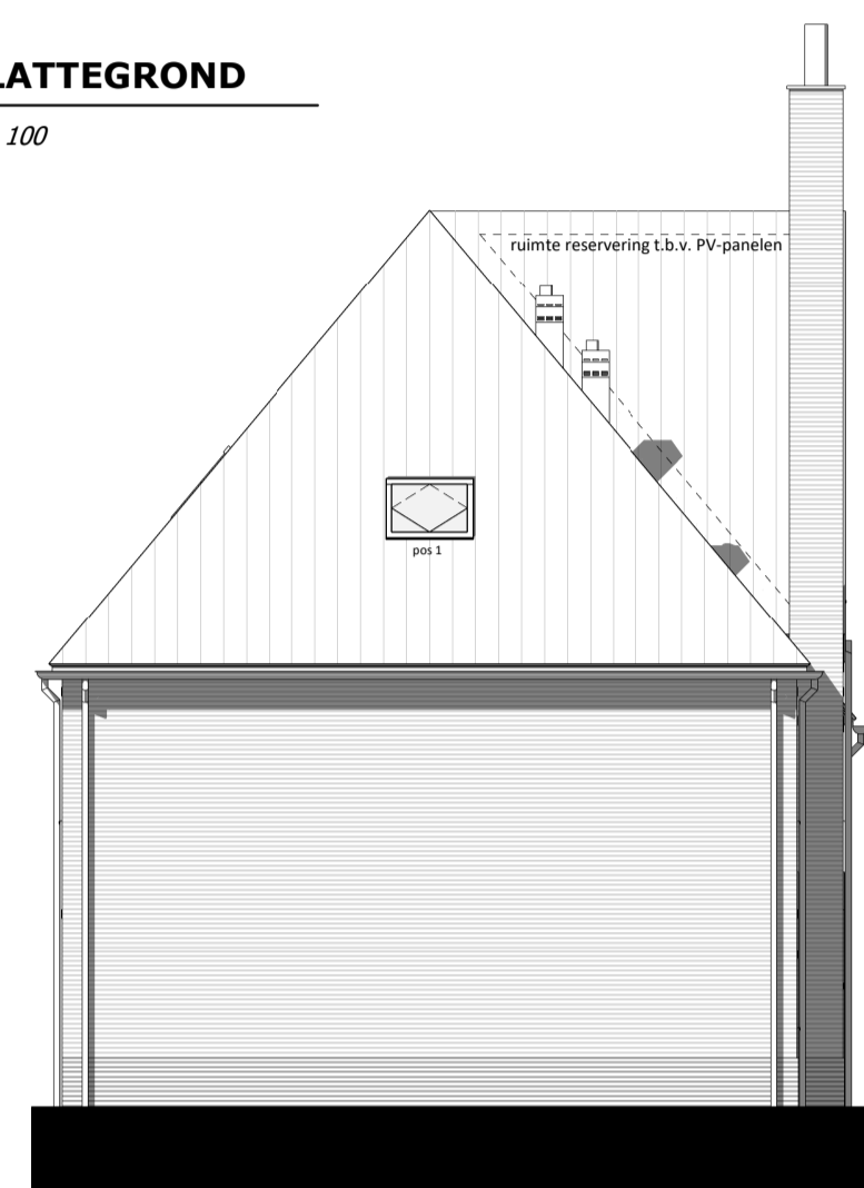
KOP GEVEL 1 : 100
