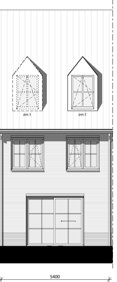
ACHTERGEVEL 1 : 100
