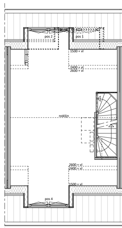
PLATTEGROND 1 : 100
