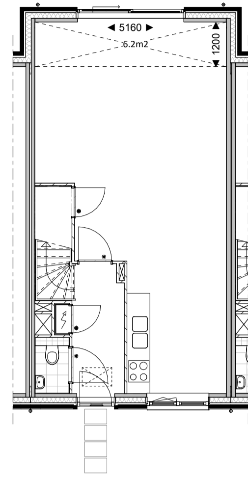
PLATTEGROND 1 : 100
