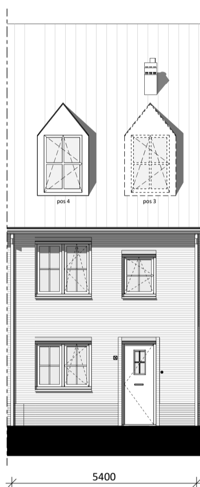
VOORGEVEL 1 : 100
