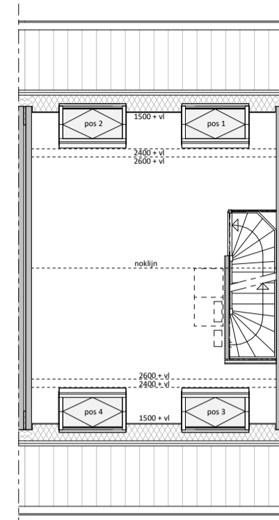
PLATTEGROND 1 : 100
