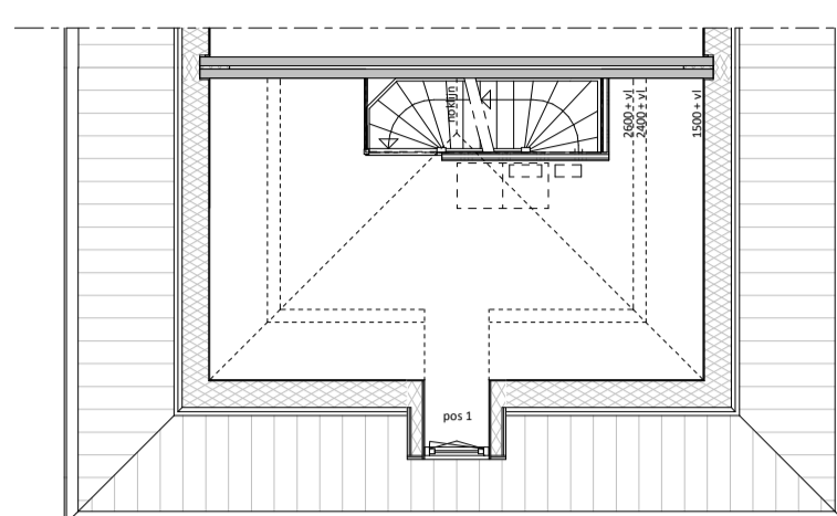
PLATTEGROND 1 : 100
