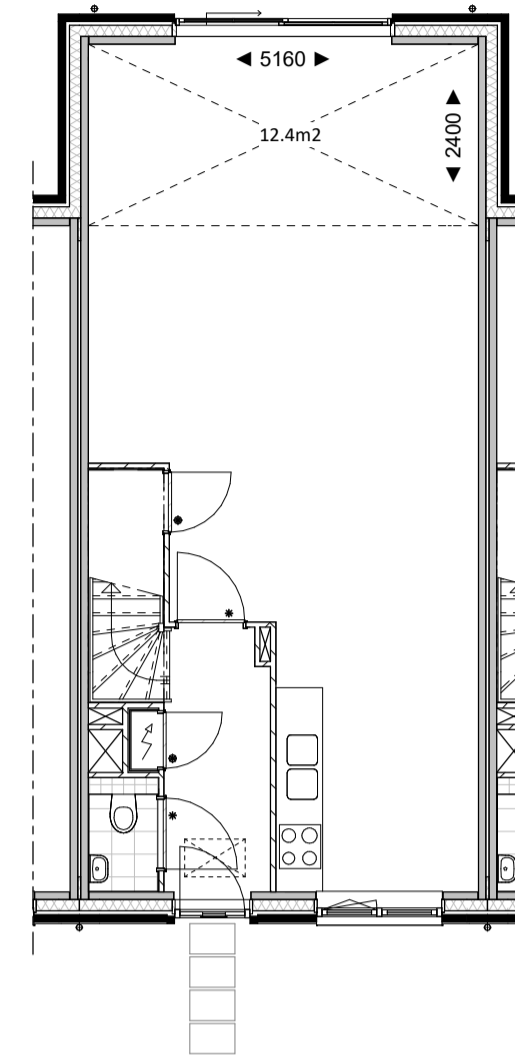
PLATTEGROND 1 : 100
