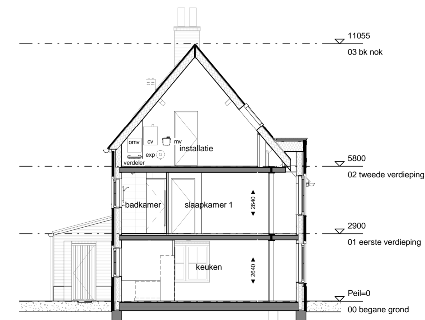
DOORSNEDEN bnr.074 1 : 100
