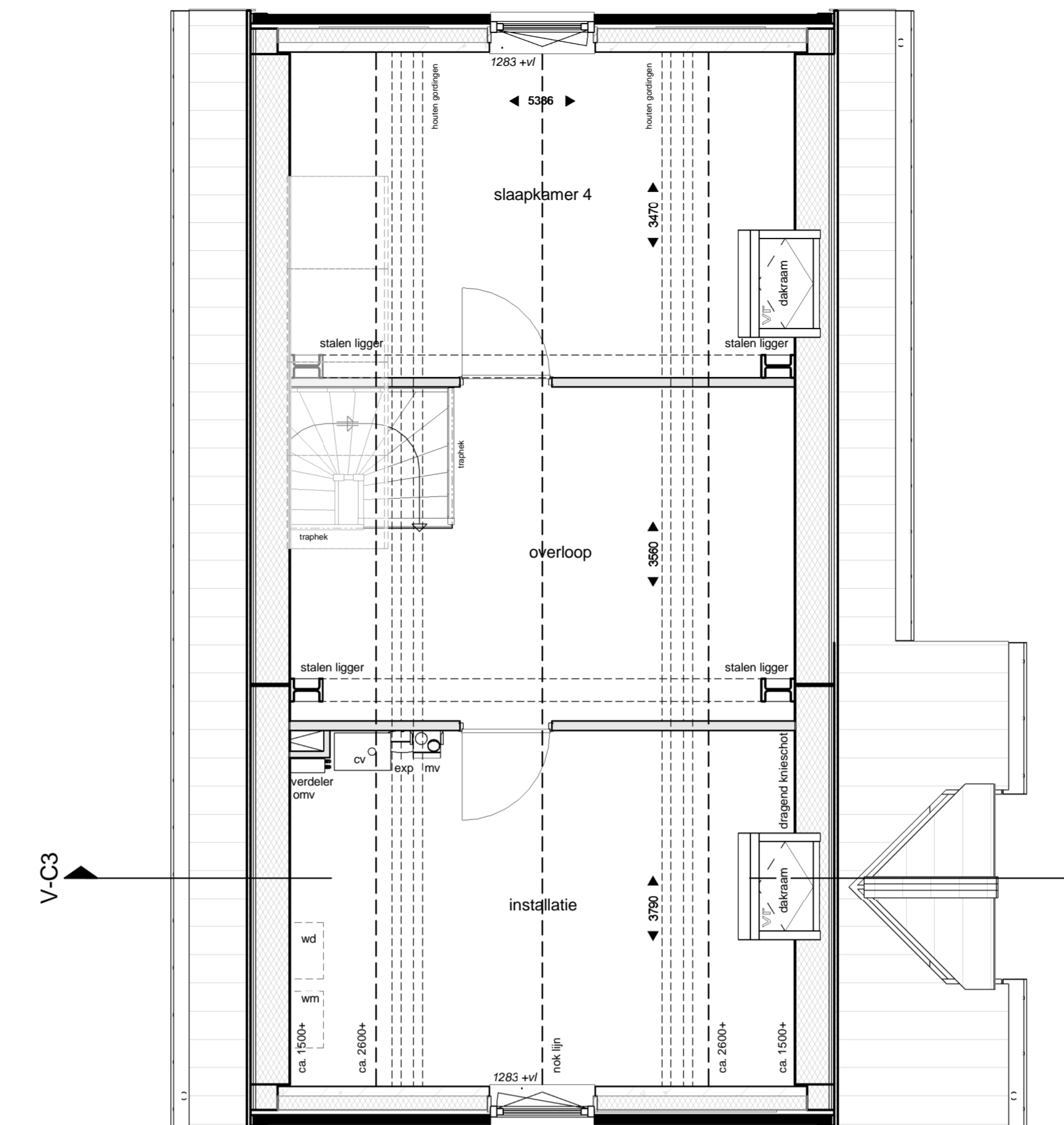
TWEDE VERDIEPING 1 : 50
