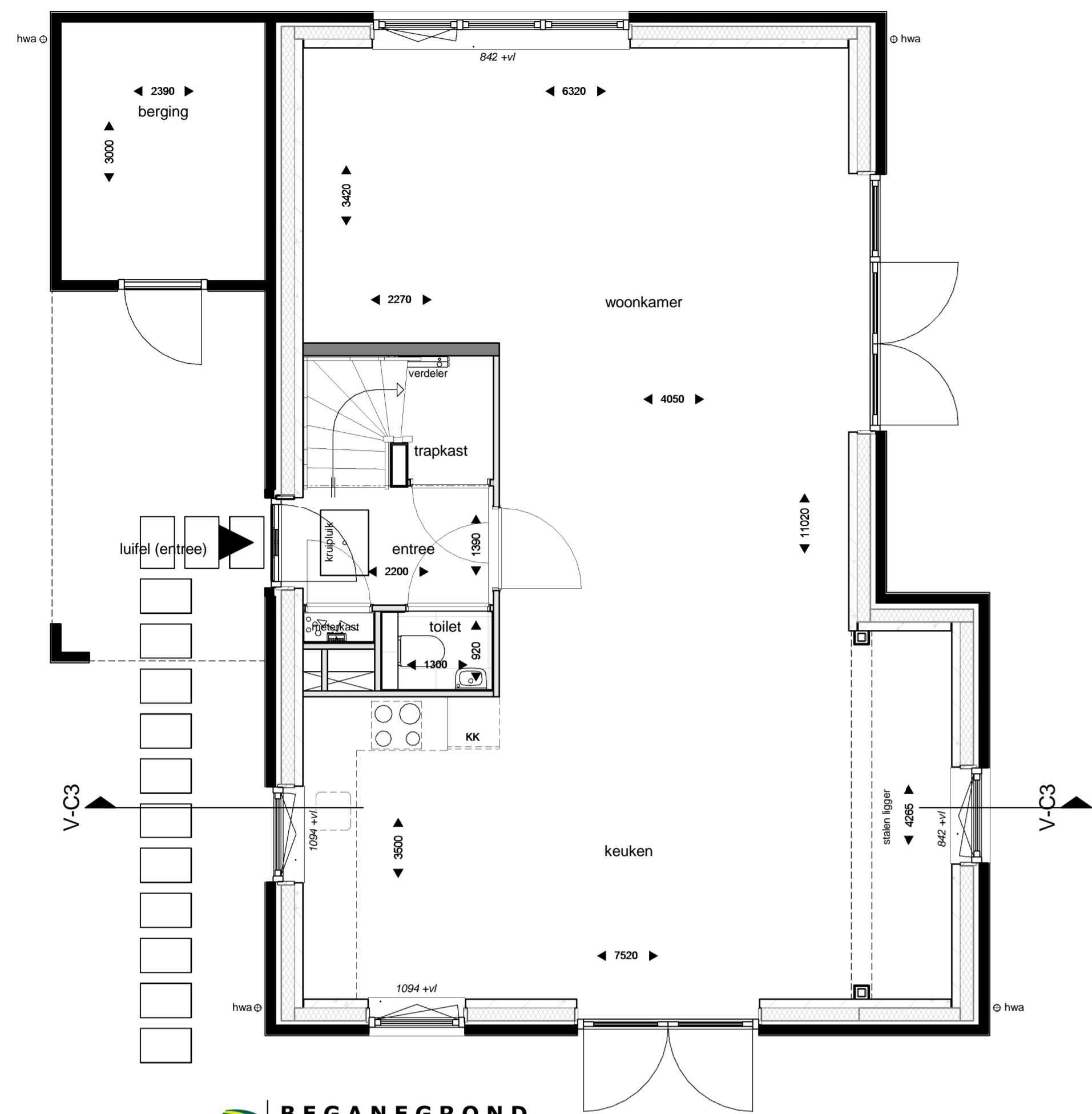
BEGANEGROND 1 : 50
